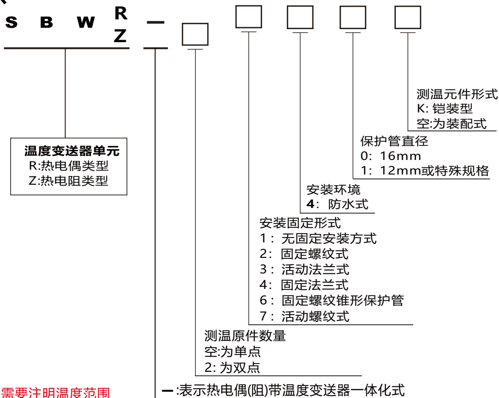
带热电偶温度变送器规格表
